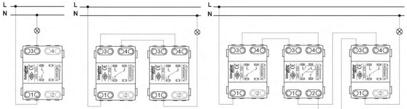
Egypólusú kapcsoló
