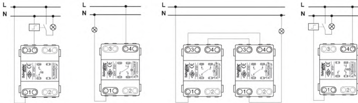
Egypólusú nyomó
