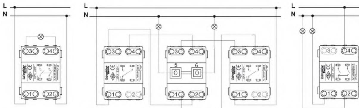
Kétpólusú kapcsoló
